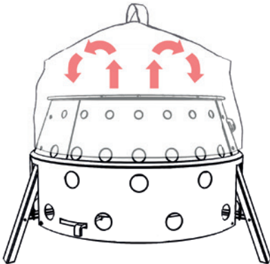
Abbildung 1: Umluftkuppel mit Atago / Funktionsprinzip
